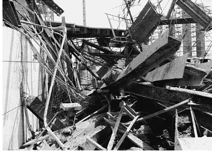
図1.1.1 支柱の座屈による倒壊の例
