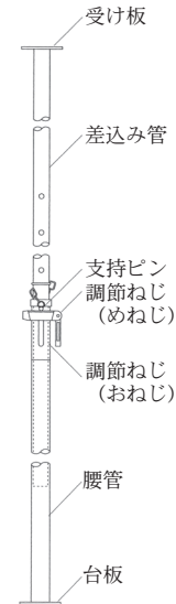
図－１ パイプサポートの例
