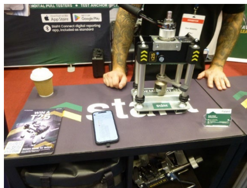
写真 12 壁つなぎの引張強度試験機の紹介
